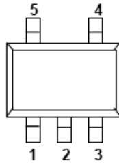
SOT-23-5/ SC-70-5
